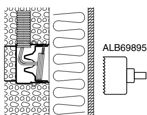
Percement du doublage ø 67 mm
