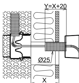
Montage du tube de raccordement, ICTA ø 25 mm
