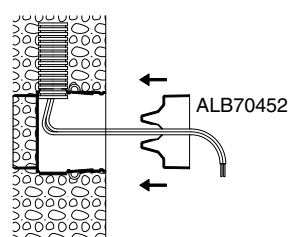
Montage du couvercle dans la boîte Préfal
