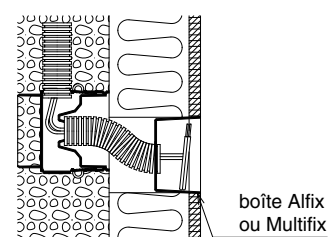
Montage de la boîte bleue
